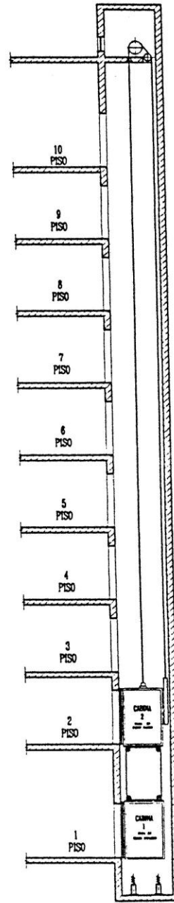
ASCENSOR MULTICABINA ESC. 1 50
